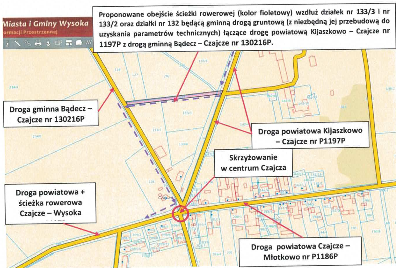
Rys. Propozycja łącznika drogowego wraz z ewentualnym obejściem ścieżką rowerową skrzyżowania w miejscowości Czajcze.
